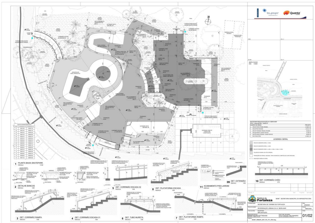
Imagem 04 – Planta 01/02 aonde podemos ver todo o skate plaza . Fonte: COPROJ/SEINF
